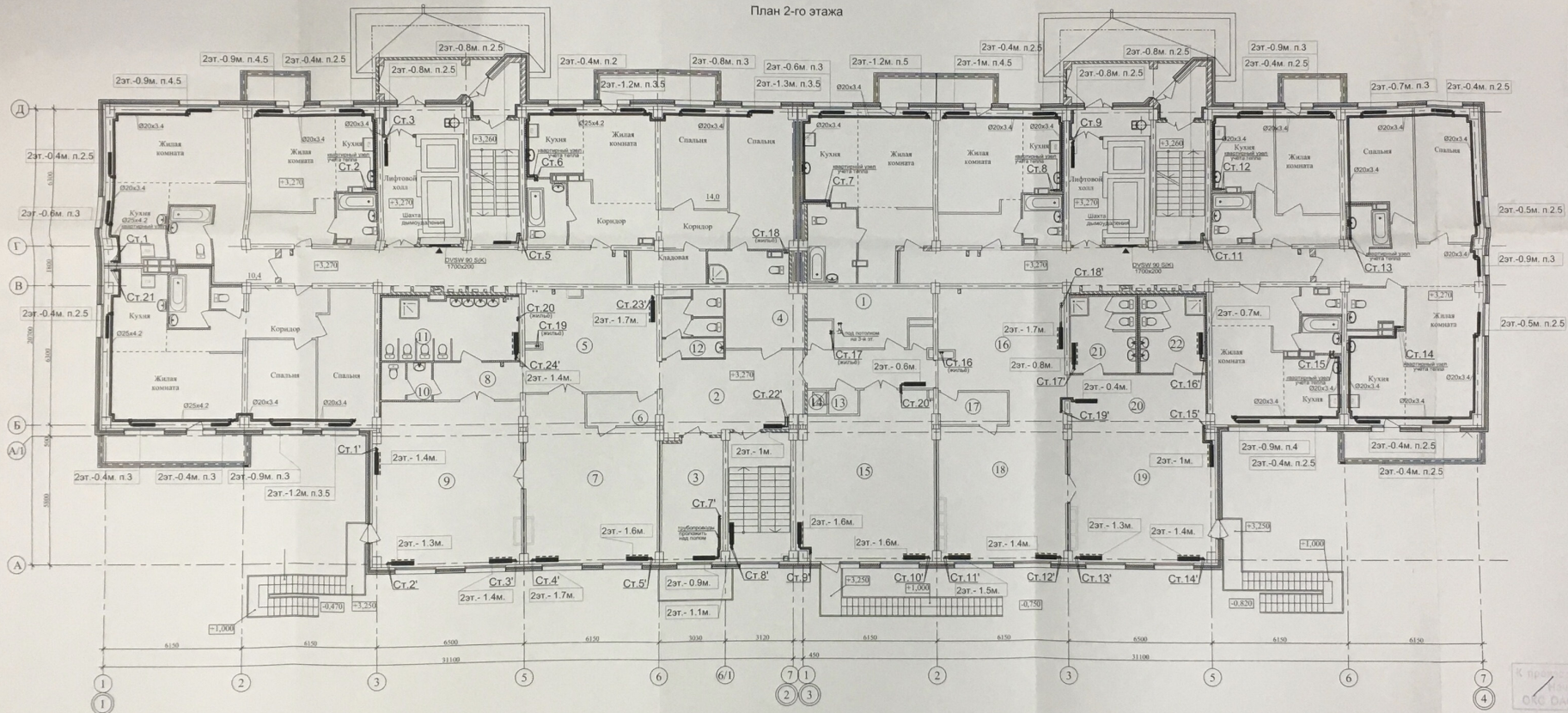
План 2-го этажа
