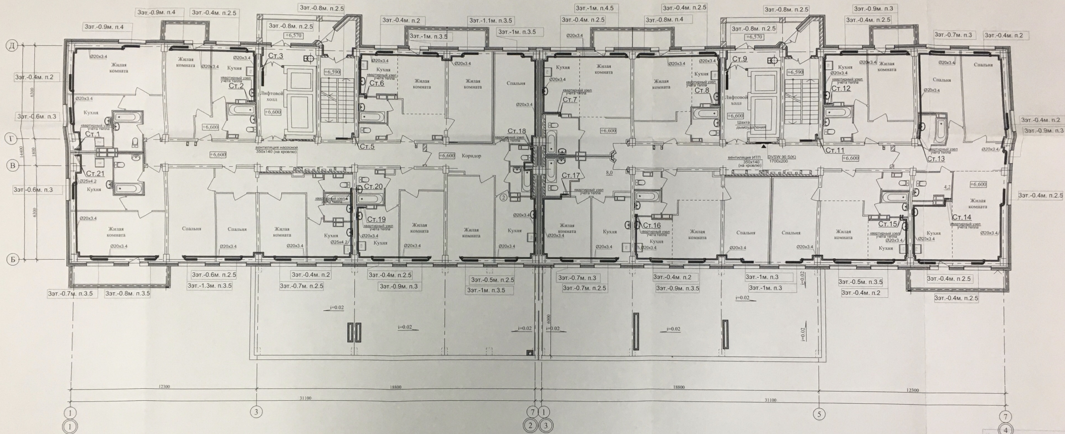
План 3-го этажа
