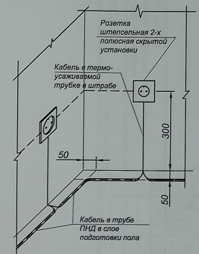
Схема расположения розеток на кухне (в зоне кухонного гарнитура)
