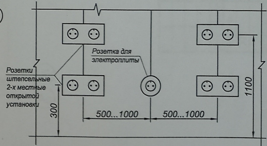
Схема расположения розеток на кухне (в зоне кухонного гарнитура)
