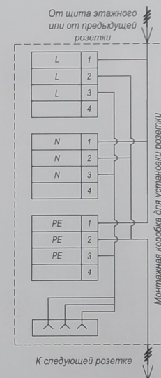
Схема расключения кабелей розеточной сети
