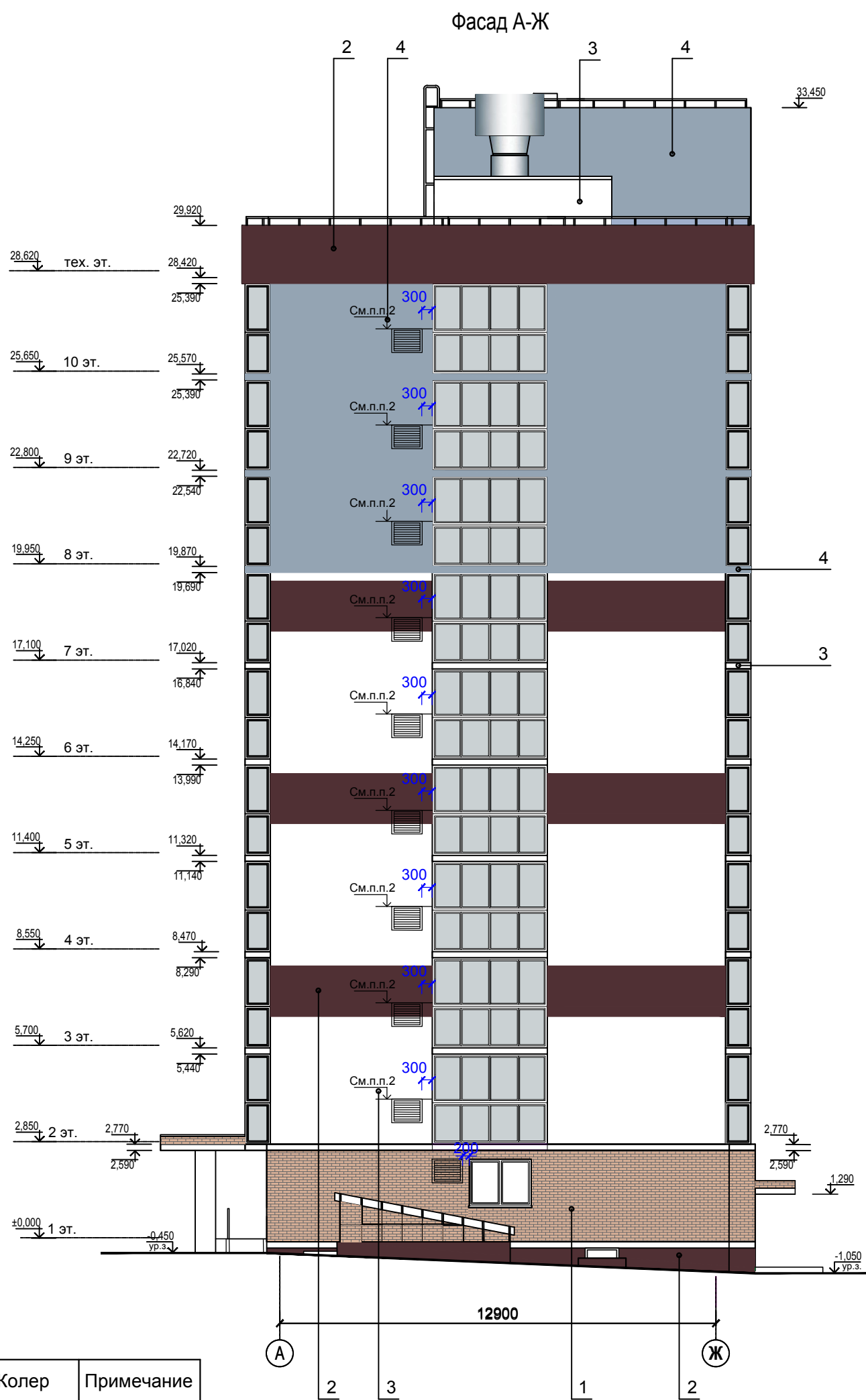
Ведомость отделки фасадов
